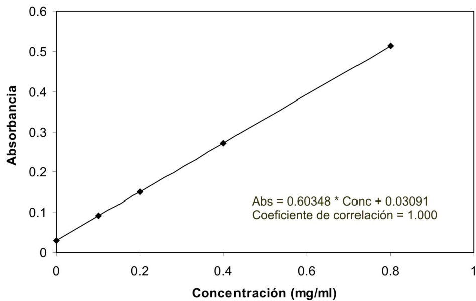
Figura 3.3: Curva de calibración
