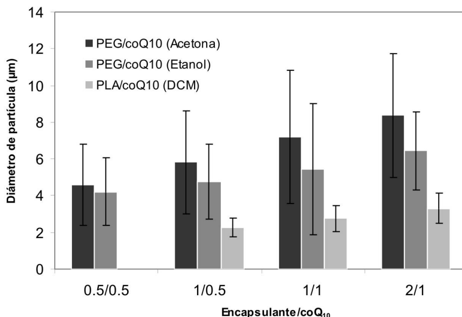
Figura 4.22: Efecto del cosolvente en el tamaño de partícula
